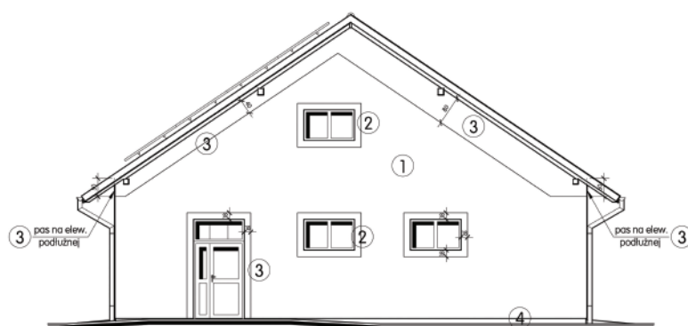
ELEWACJA WSCHODNIA
