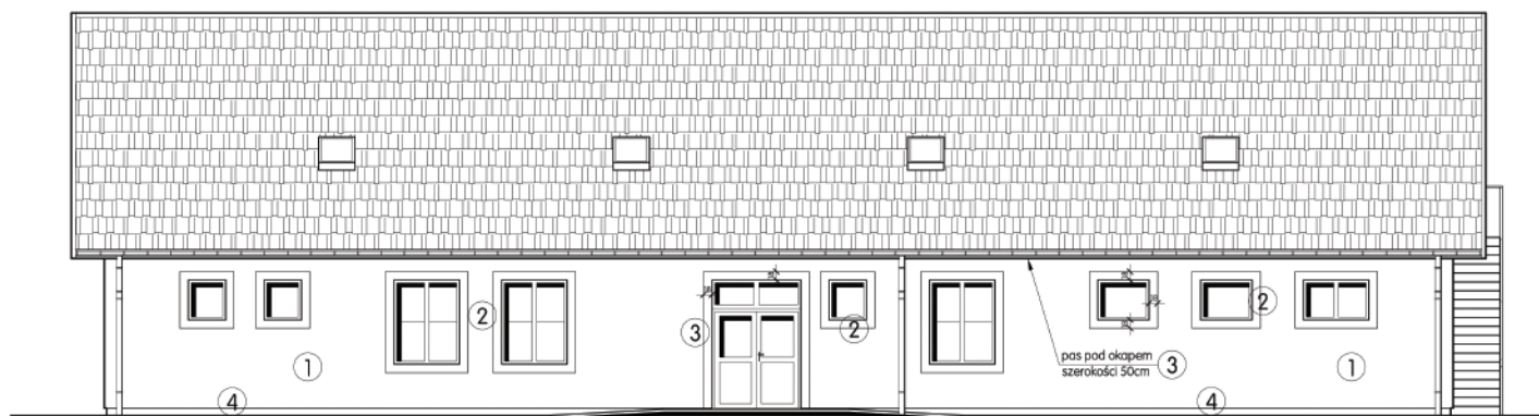
ELEWACJA PÓŁNOCNA
